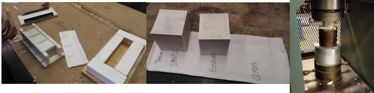
写真3 コンクリートキューブの製作と試験の様子
